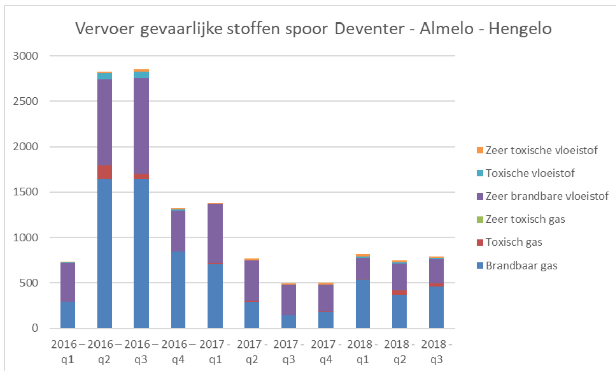
Figuur 1: Aantal gevaarlijke stoffen per kwartaal in ketelwagenequivalenten op traject Deventer - Almelo - Hengelo
